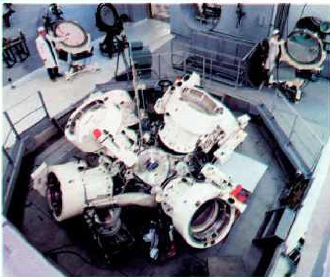
Циклотрон У-240
