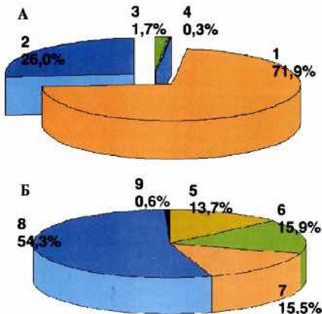
Рис. 4. Вклад различных источников ионизирующего излучения в общую дозовую нагрузку населения: а) от всех источников: 1-естественные источники; 2-медицинские процедуры; 3-радиоактивные осадки, последствия ядерных взрывов в атмосфере; 4- атомная энергетика; б) только от естественных источников: 5-космическое излучение; 6-излучение горных пород и материалов; 7-излучение продуктов питания и напитков; 8-радон и продукты его распада; 9-прочие источники.
