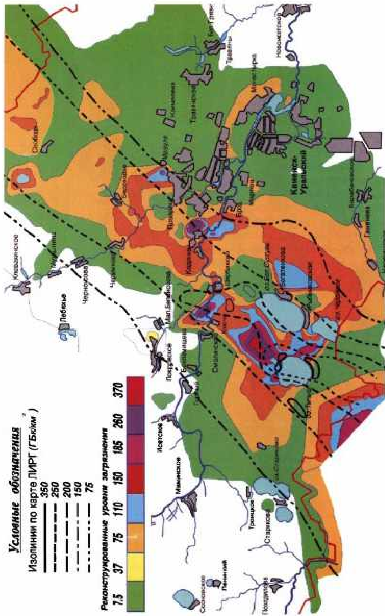
Рис.30. Схема распределения стронция-90 на территории Каменского района Свердловской области по данным ЛИРГа (1958г.) и результатам реконструкции измерений ИПЭУРО РАН в 1993г.
