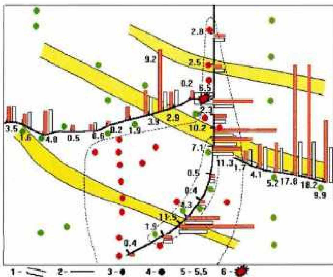
Рис.23. Характеристика района ядерных взрывов "Грифон" на Осинском нефтяном месторождении: 1-локальные разломы земной коры; 2-профили измерений; 3-скважины с концентрацией цезия-137 в воде более 50 Бк/л; 4-скважины с концентрацией цезия в воде менее 50 Бк/л; 5-концентрация радона в почвенном воздухе, кБк/м 3 ; 6-место проведения ядерных взрывов
