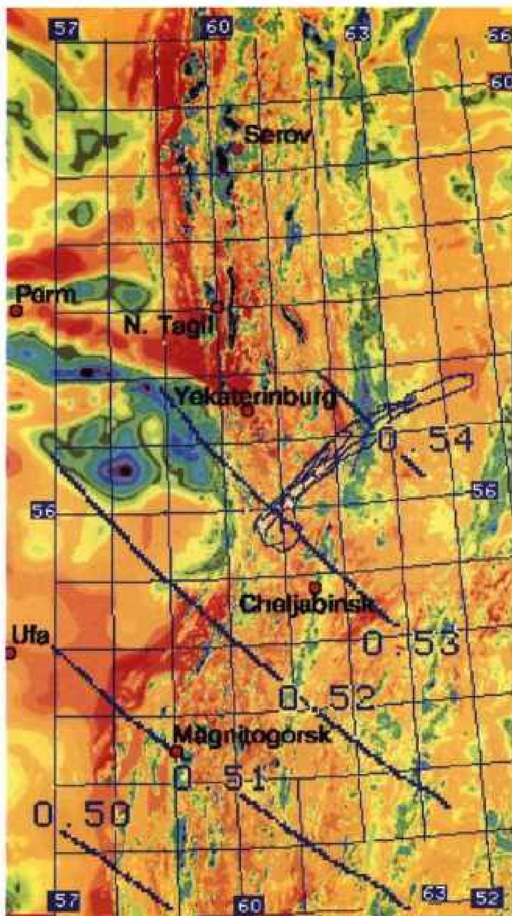
Рис.28. Карта - схема формирования радиоактивного облака взрыва магнитным полем Земли. Синими линиями выделено главное магнитное поле, растушевкой - аномальное магнитное поле. Синим цветом обозначены высокие значения поля ( 0,02 - 0,05 эрстеда)
