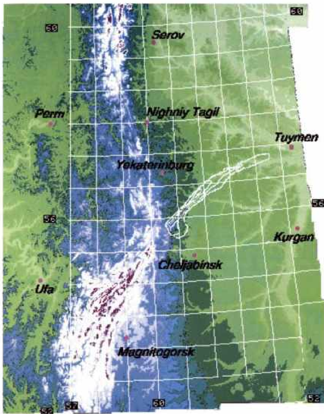
Рис.27. Схема формирования направления ветра в период аварии на ПО МАЯК. Темным цветом выделены повышенные участки рельефа
