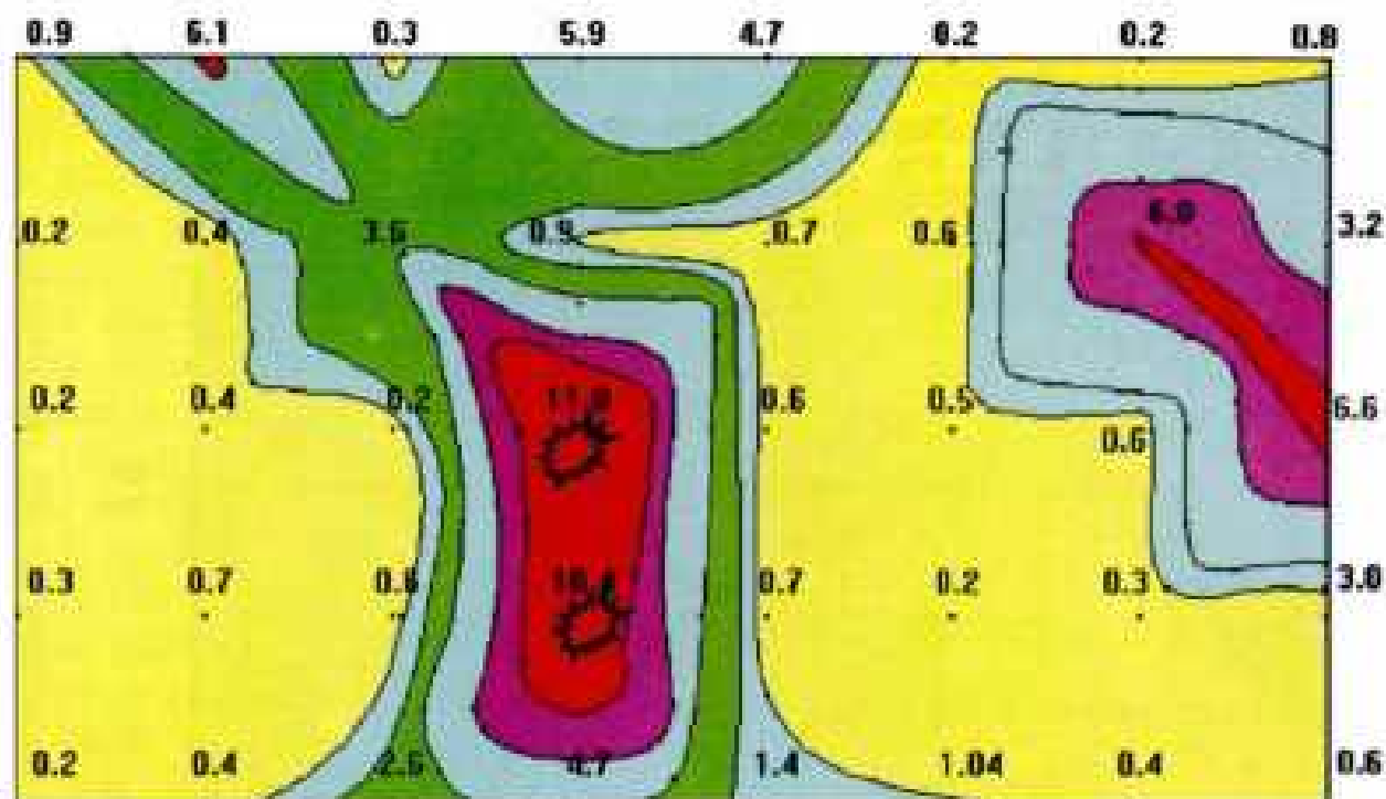
Рис.22. Распределение концентрации радона в почвенном воздухе (кБк/м 3 ) вокруг скважин на Осинском месторождении нефти. Звездочками отмечены места взрывов
