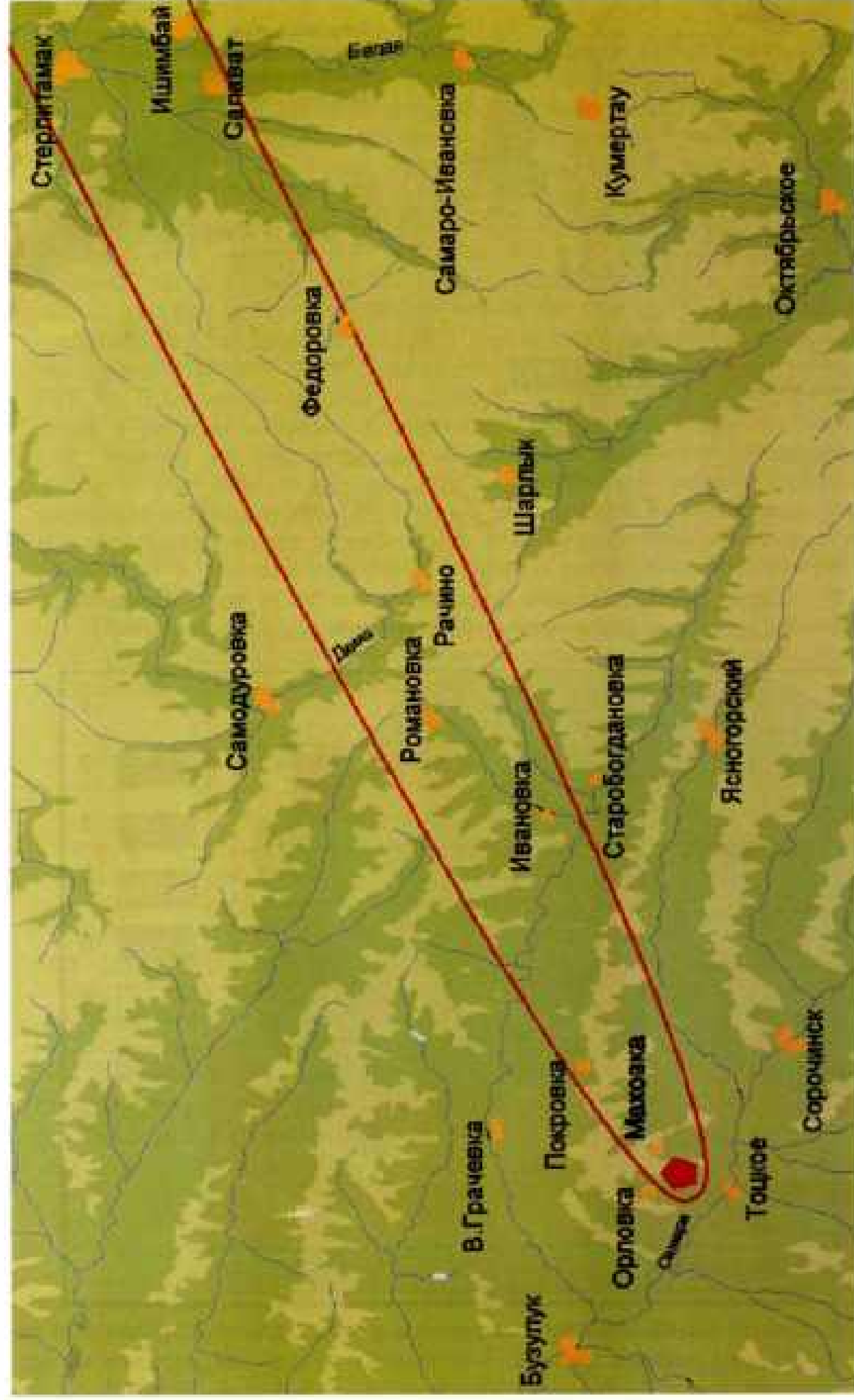
Рис.21. Схема предполагаемого распространения радиоактивного облака после взрыва атомной бомбы во время Тоцких учений (модель 1998г.)
