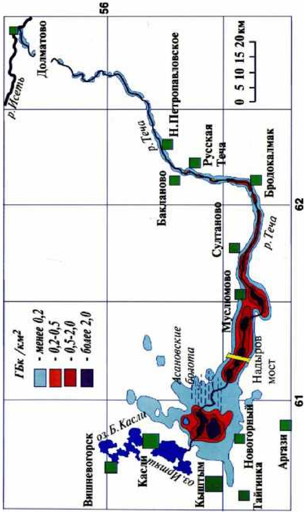
Рис.17. Концентрация цезия-137 в донных отложениях р. Течи
