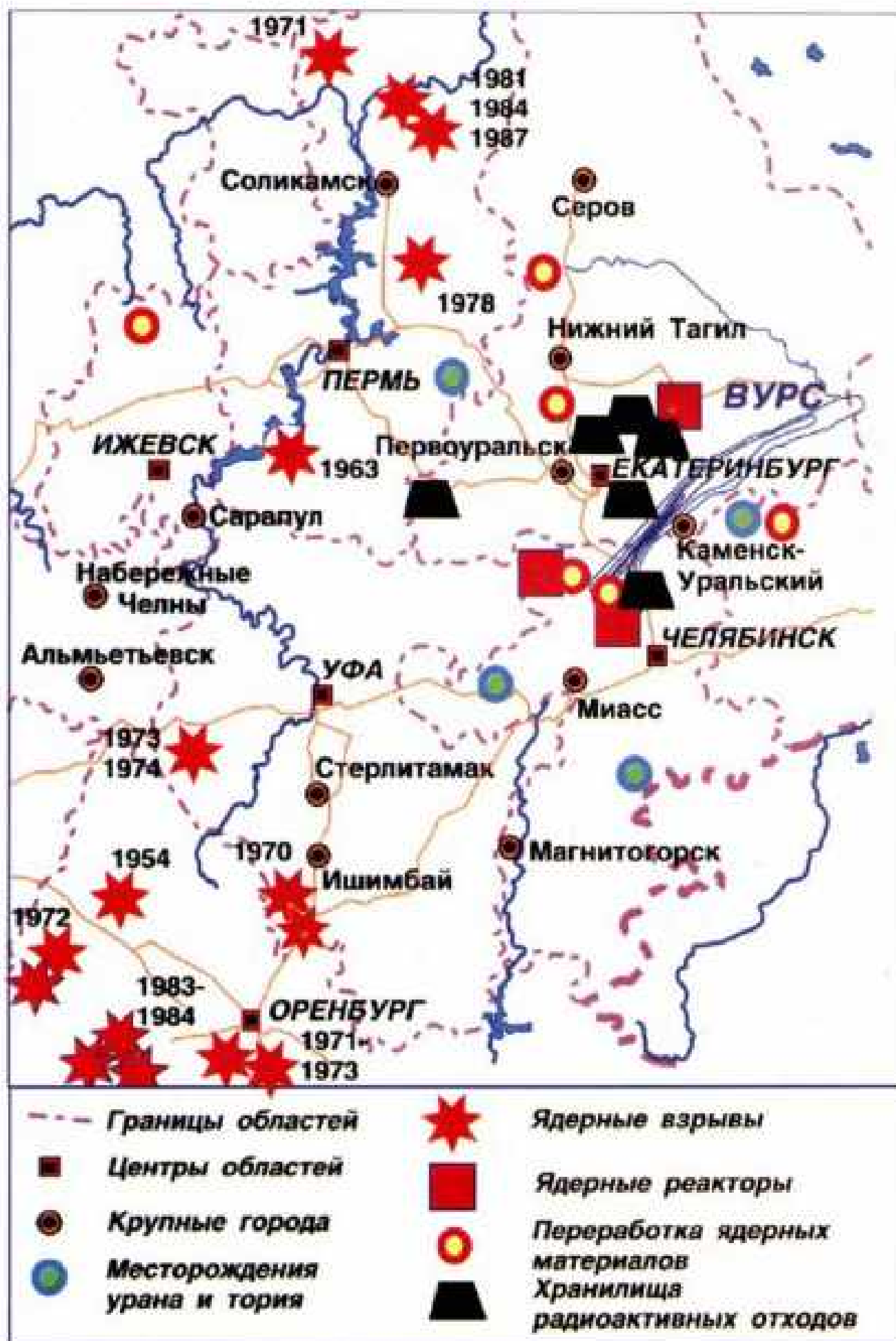
Рис.7. Схема расположения предприятий ядерно-топливного цикла в Уральском регионе
