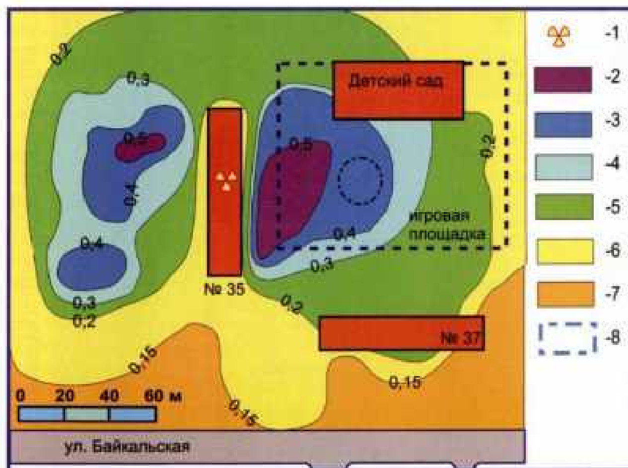
Рис.20. Схема интенсивности гамма-поля от источника, расположенного на чердаке жилого здания: 1-источник цезия-137; мощность экспозиционной дозы: 2 - более 0,5 мкЗв/ч; 3 - 0,5-0,4; 4 - 0,4-0,3; 5 - 0,3-0,2; 6 - 0,2-0,15; 7-менее 0,15 мкЗв/ч; 8- территория детского сада
