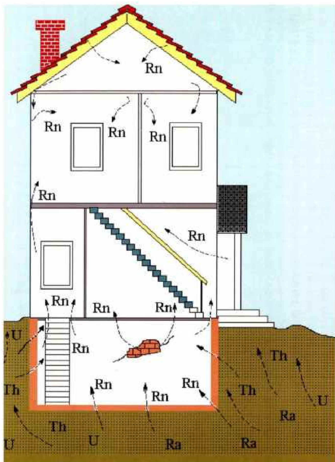
Рис.14. Пути попадания радона из почвы и строительных конструкций в жилище
