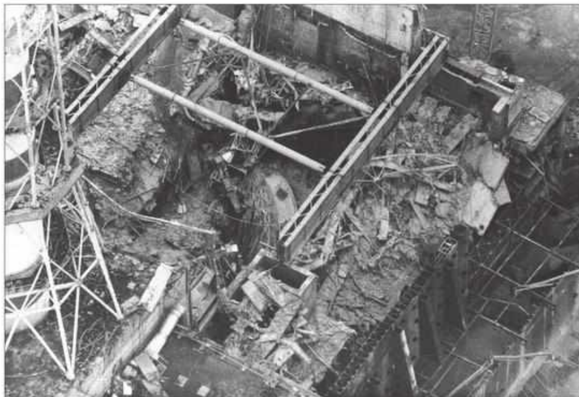
Балка «Самолет» установлена, внизу видна перевернутая крышка реактора «Елена». 23 сентября 1986 г.
