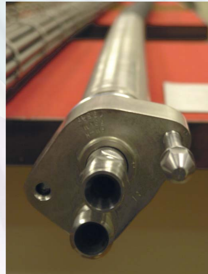
Детали тепловыделяющих элементов для первой в мире АЭС, изготовленные на заводе № 12, 1954 г.
