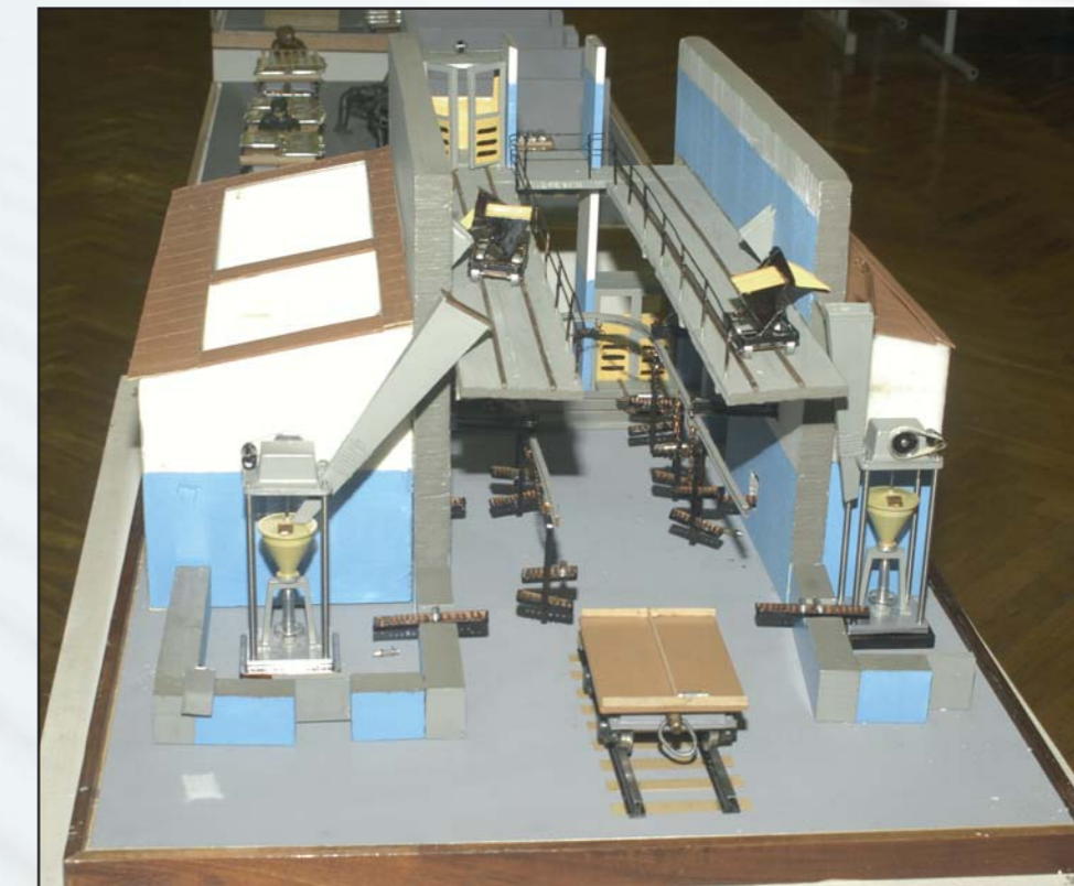
Макет-реконструкция техпроцесса.
