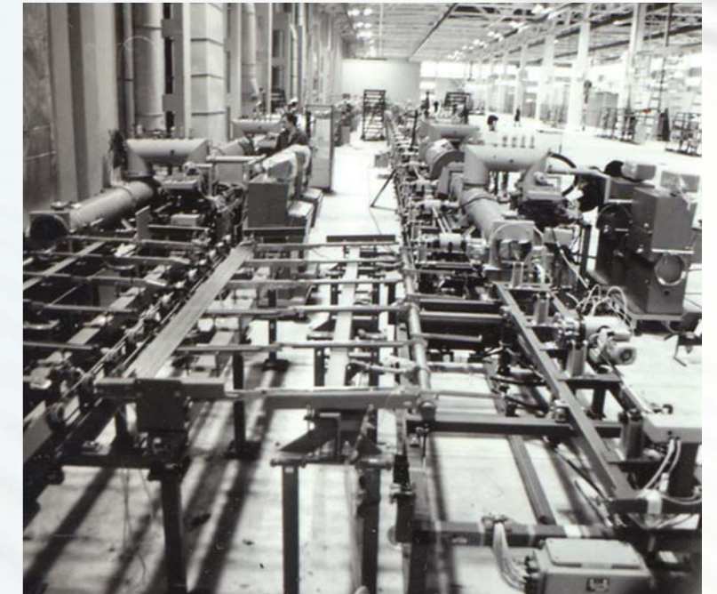
Обсуждение хода внедрения модульной линии изготовления твэлов по проекту Германской Демократической Республики.
