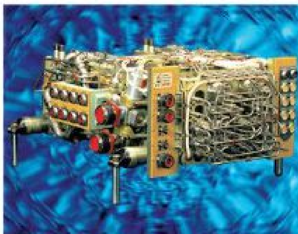
Электрохимический генератор «Фотон»
