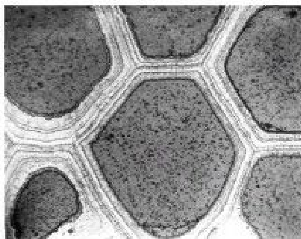
Структура кермета на основе металлической матрицы и топливных частиц
