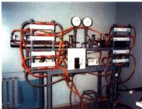
Макетная установка на основе металлгидридных насосов для генерации холода
