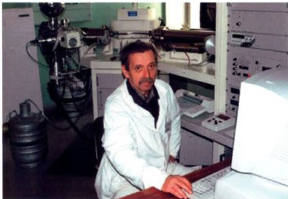
Руководитель группы Ефремов Ю.П. проводит измерения изотопного состава ЯМ на масс-спектрометре МАТ-262
