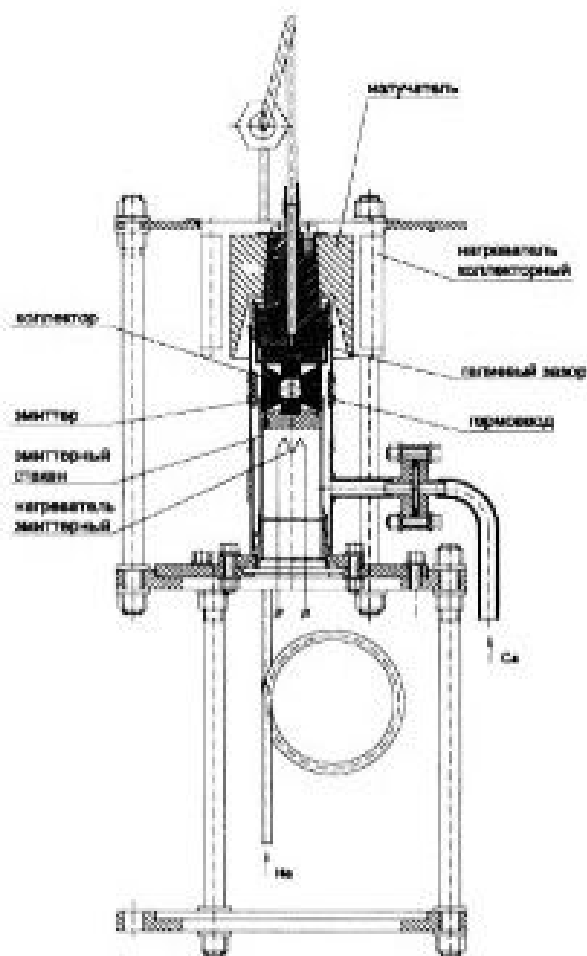
Конструктивная схема ТЭП с малым зазором
