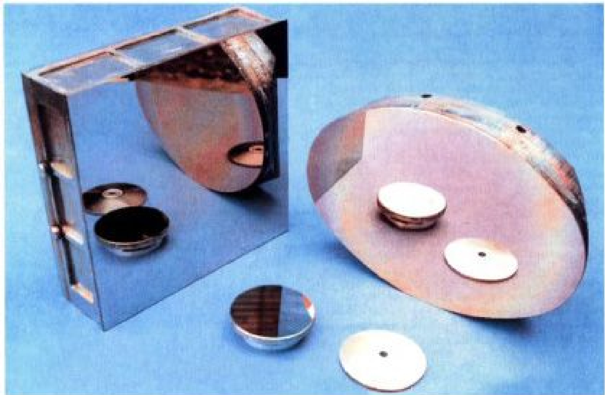
Внешний вид охлаждаемых зеркал для мощных лазеров
