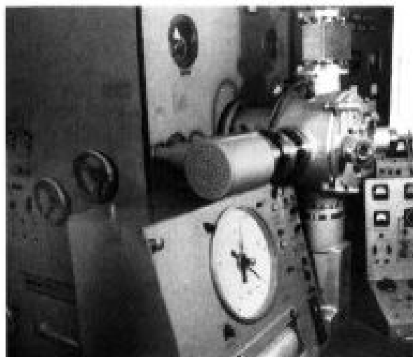
Электроно-лучевая установка для определения прочности при высоких температурах вплоть до 3000 К
