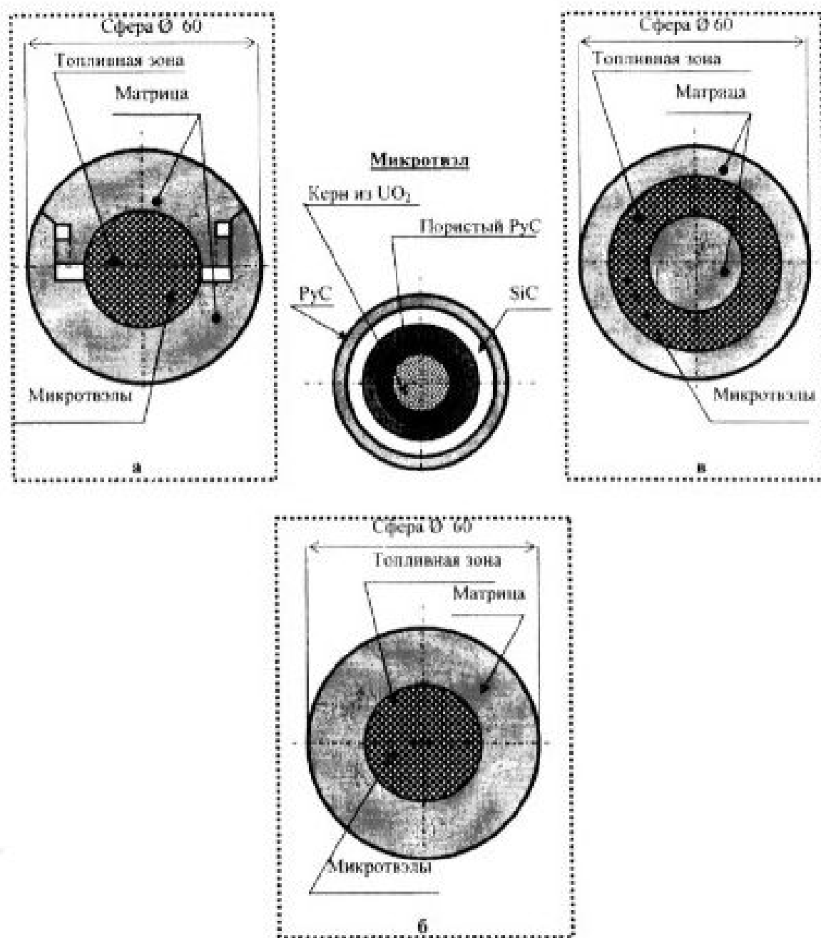
Шаровые уран-графитовые твэлы ВТГР: а — сборный, б — монолитный двухзонный, в — монолитный трехзонный
