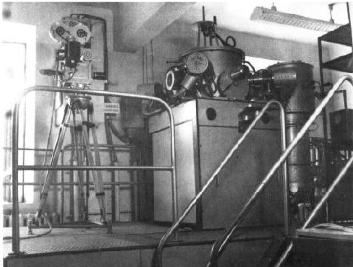
Установка с четырьмя электродными пушками для определения термopочности при различных скоростях нагрева до высоких температур вплоть до 3000 К
