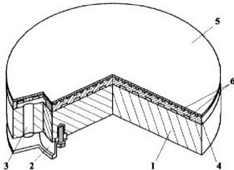
Конструкция охлаждаемых изделий металлооптики для мощных лазеров 1 — основа зеркала, 2 — элементы крепления, 3 — системы подвода и отвода охлаждающей жидкости, 4 — промежуточная пластина, 5 — зеркальная пластина, 6 — каналы охлаждения
