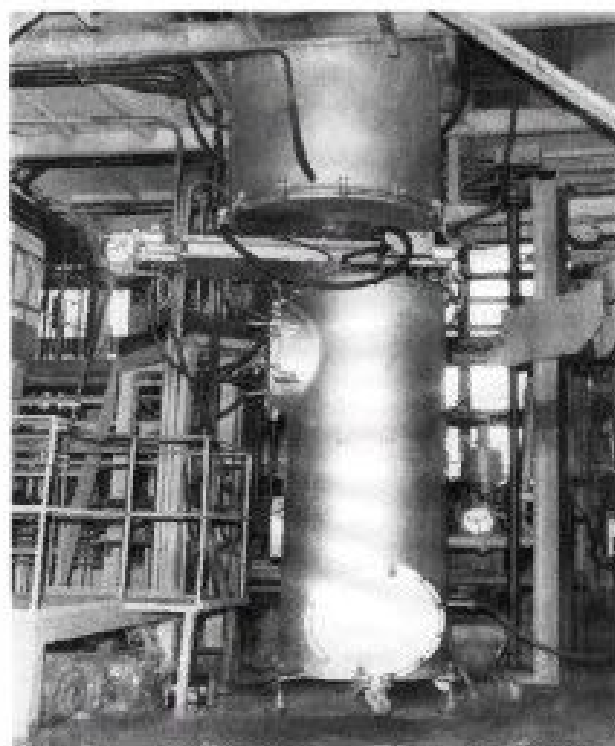
Вакуумная до (2200 °С) электропечь с форкамерой
