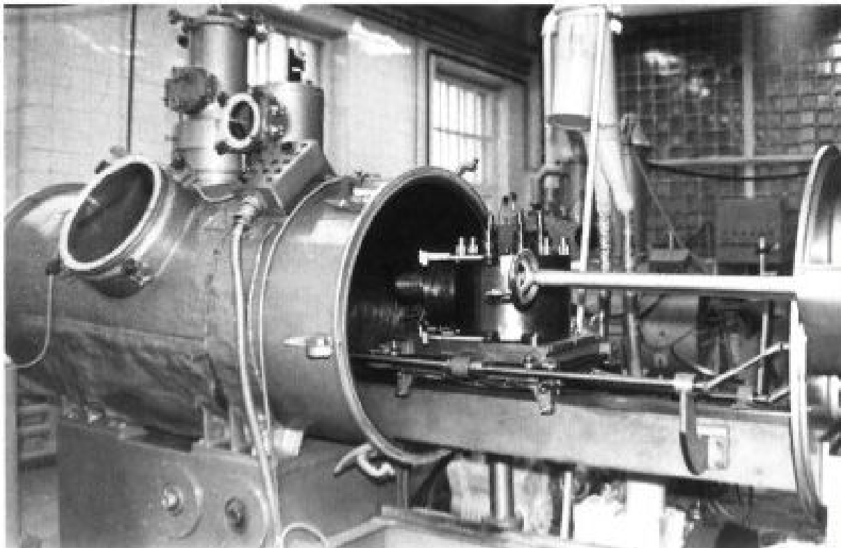
Установка для нанесения покрытий плазменным напылением
